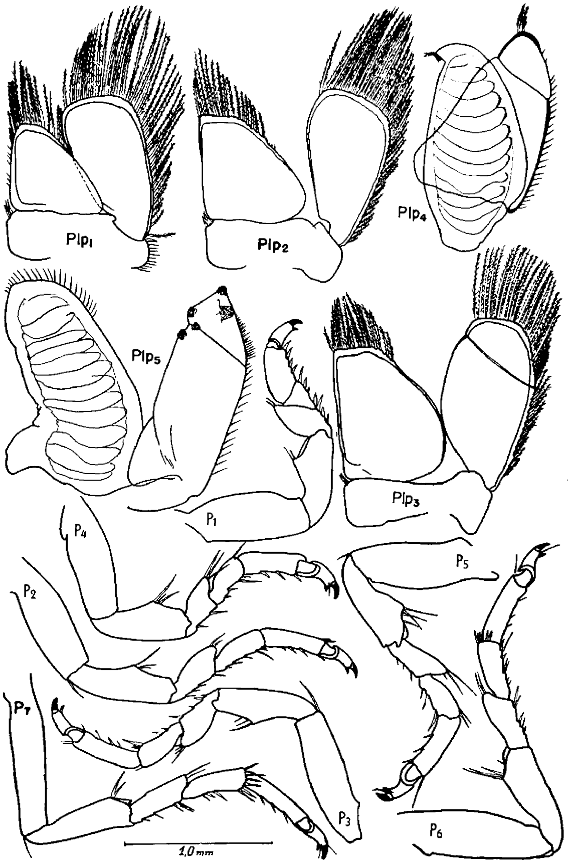
Fig. 13, Cymodoce barrerae (Boone, 1919). Pip1 a Pip5, primeiro ao quinto pleópodo. P1 a P7, primeiro ao sétimo pereópodo.
