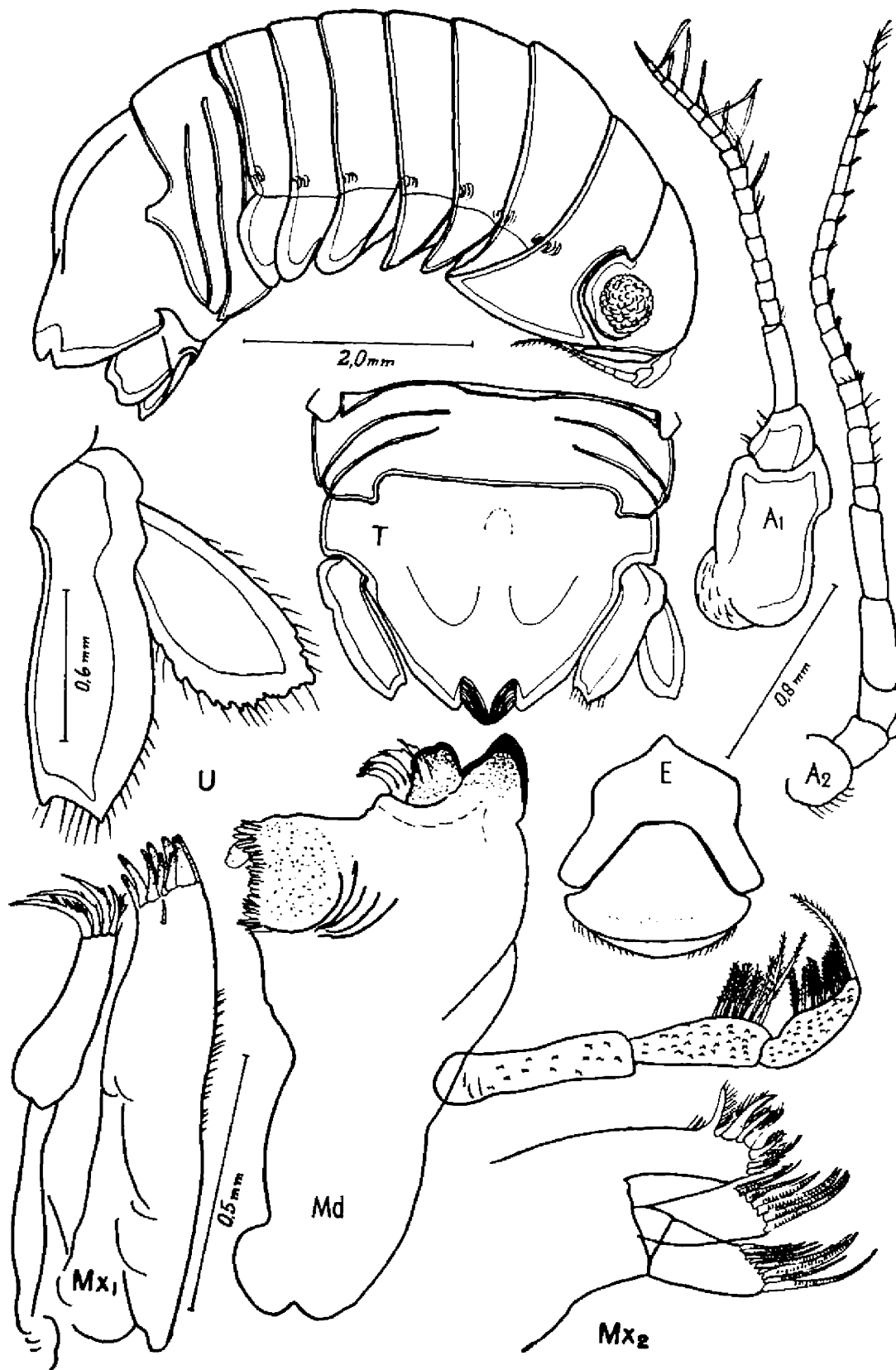
Fig. 12. Cymodoce barrerae (Boone, 1919). Fêmea em vista lateral. T, abdome e urópodos. A1 e A2, primeira e segunda antena. U, urópodo. Mx1 e Mx2, primeira e segunda maxila. Md, mandíbula. E, epistoma e lábio superior.
