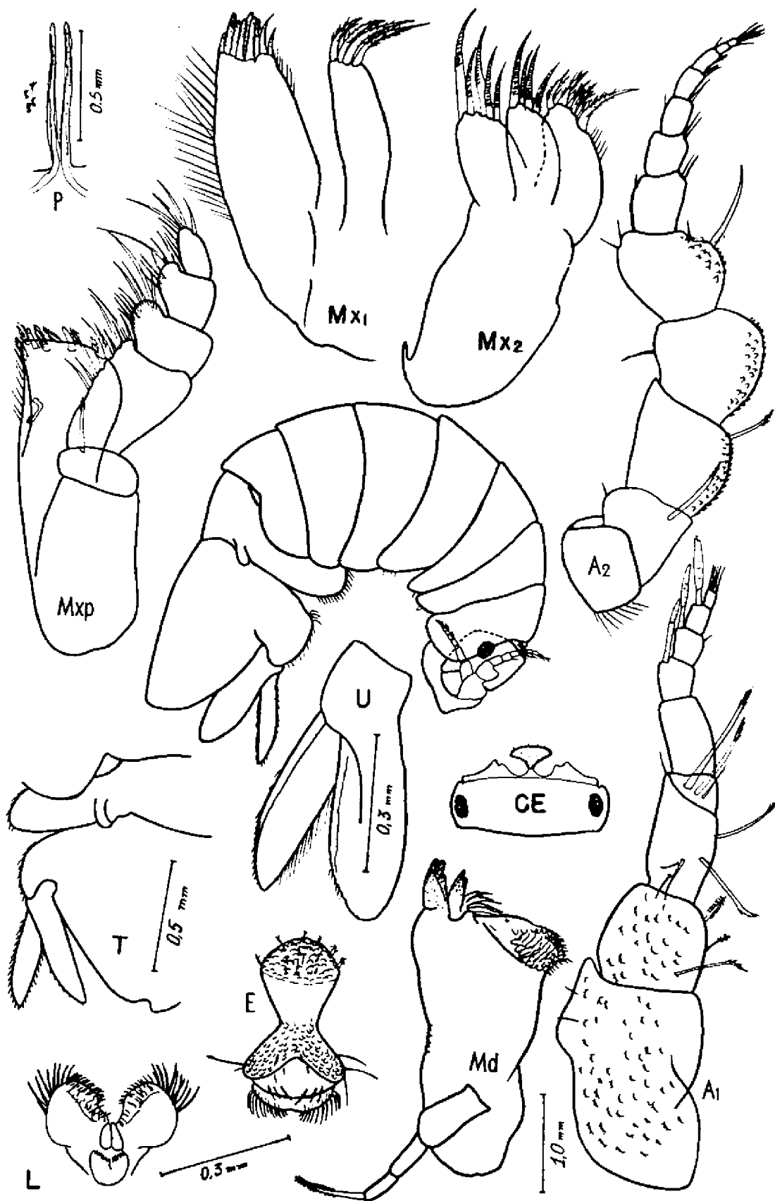
Fig. 18, Pseudosphaeroma rhombofrontale (Giambliagi, 1922). Macho em vista lateral. P, pênis. Mx1 e Mx2, primeira e segunda maxila. A1 e A2, primeira e segunda antena. Mxp, maxilípede. T, abdome e urópodo em vista parcial para mostrar as margens látero-posteriores do télson um pouco encurvadas. U, urópodo. CE, cabeça e epístoma em vista dorsal. L, lábio inferior. E, epístoma e lábio superior. Md, mandíbula.
