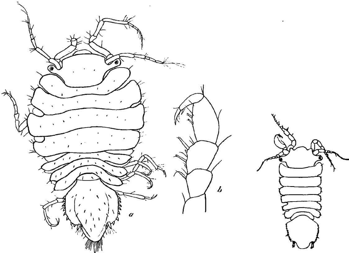
Abb. 105. Paramunna kerguelensis n. sp. a ( \times 54 ), b Greiffuß ( \times 93 ). Abb. 106. Paramunna capensis n. sp. ( \times 96 ).
