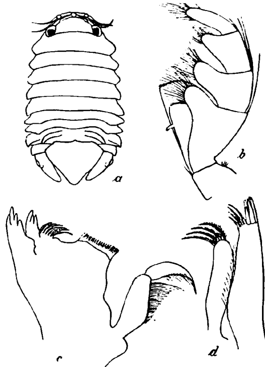
Abb. 48. Cassidinopsis maculata STUDER. a von oben ( \times 4,6 ), b Maxillarfuß, c Mandibel, d erste Maxille.
