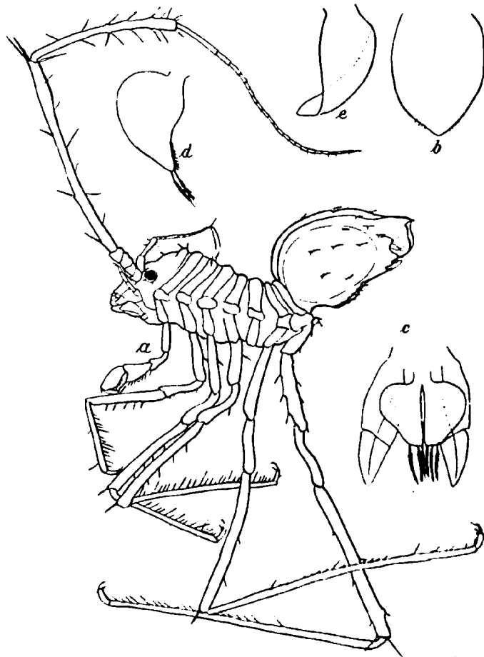
Abb. 94. Munna globicauda n. sp. a ♀ (× 10), b—e Pleopoden des ♀ (× 18).
