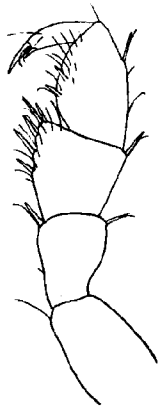
Abb. 89. Munna studeri HILGENDORF. Greiffuß des ♀.
