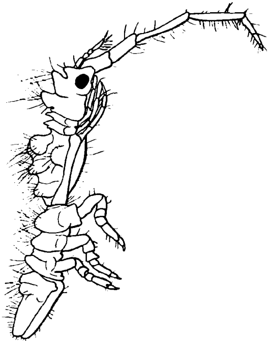
Abb. 55. Astacilla setosa n. sp. (× 16).
