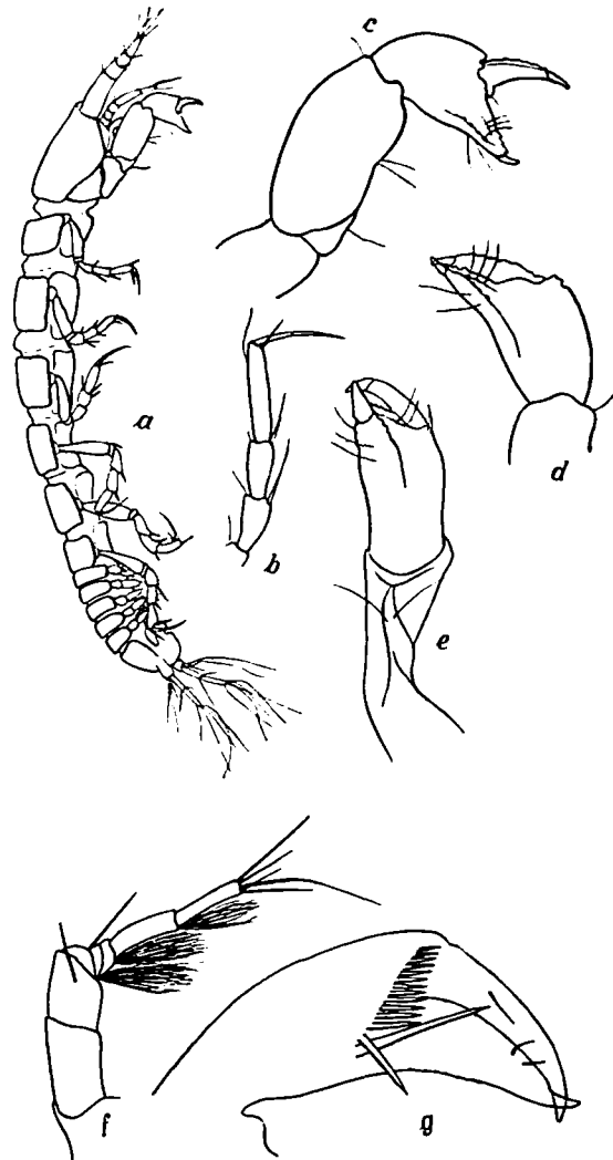
Abb. 10. Leptognathia antarctica n. sp. a ♀ (× 36). b 2. Fuß, c, d, e , Schere, f , zweite Antenne des ♂, g Schere, des ♂ von der Innenseite (× 55).
