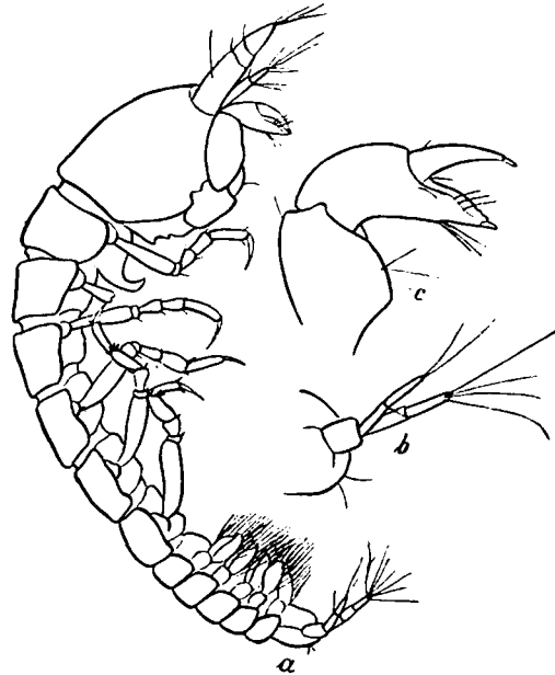
Abb. 9. Typhlotanais macrocephala HANSEN. a ♀ (× 48), b Uropod, c Schere (× 114).
