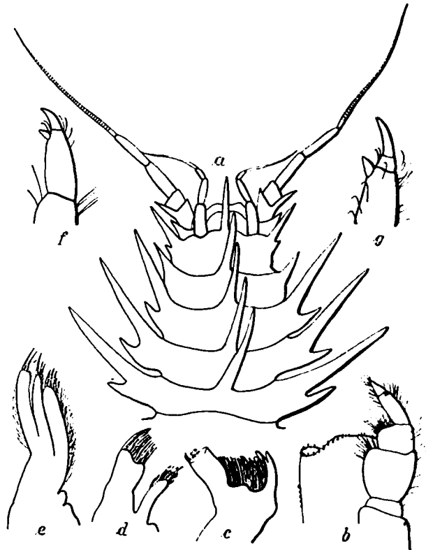
Abb. 65. Jolante acanthonotus BEDDARD. a Kopf und vordere Segmente ( \times 6 ), b Maxillarfuß, c Mandibel, d erste, e zweite Maxille ( \times 23 ), f Endglied des zweiten und g des vierten Fußes ( \times 43 ).
