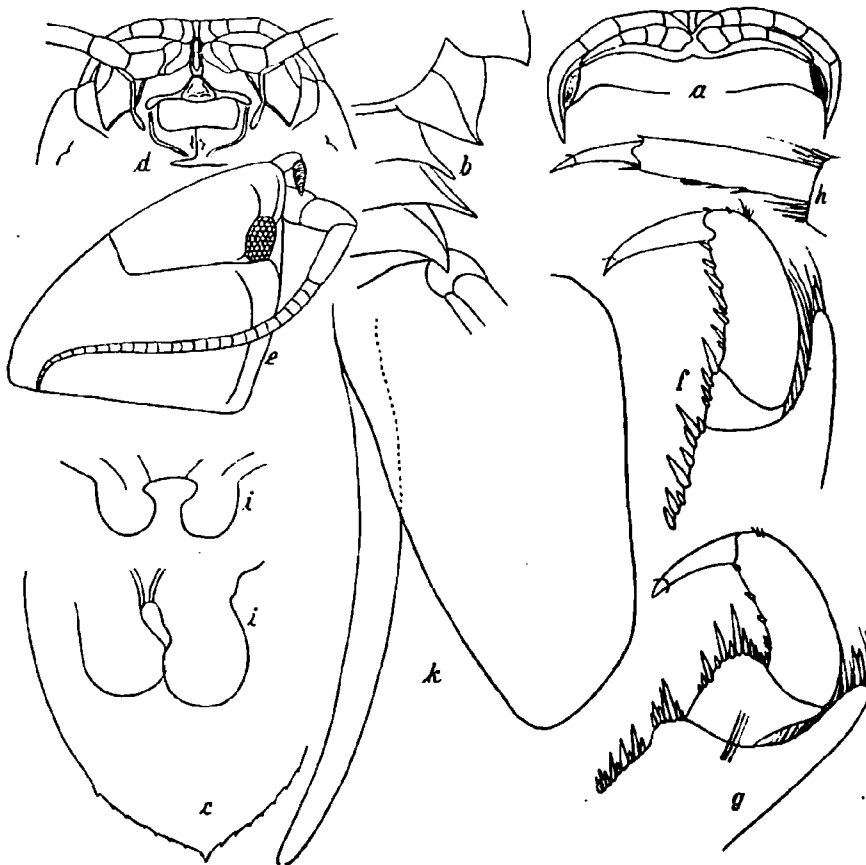
Abb. 35. Cirolana albinota n. sp. a Kopf von oben ( \times 4,5 ), b Seitenspitzen der letzten Rumpfsegmente und des Abdomens ( \times 4,5 ), c Spitze der Schwanzplatte, d Kopf von unten, e Kopf von der Seite, f erster Fuß, g zweiter Fuß, h Spitze des siebenten Fußes ( \times 18 ), i Griffler zweier Exemplare, k zweiter Pleopod des ♂ ( \times 10 ).
