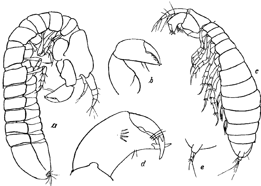
Abb. 17. Strongylura antarctica n. sp. a ♀ ( \times 36 ), b Schere stärker vergrößert, c ♂ ( \times 48 ). d Schere, e Uropod desselben, stärker vergrößert.
