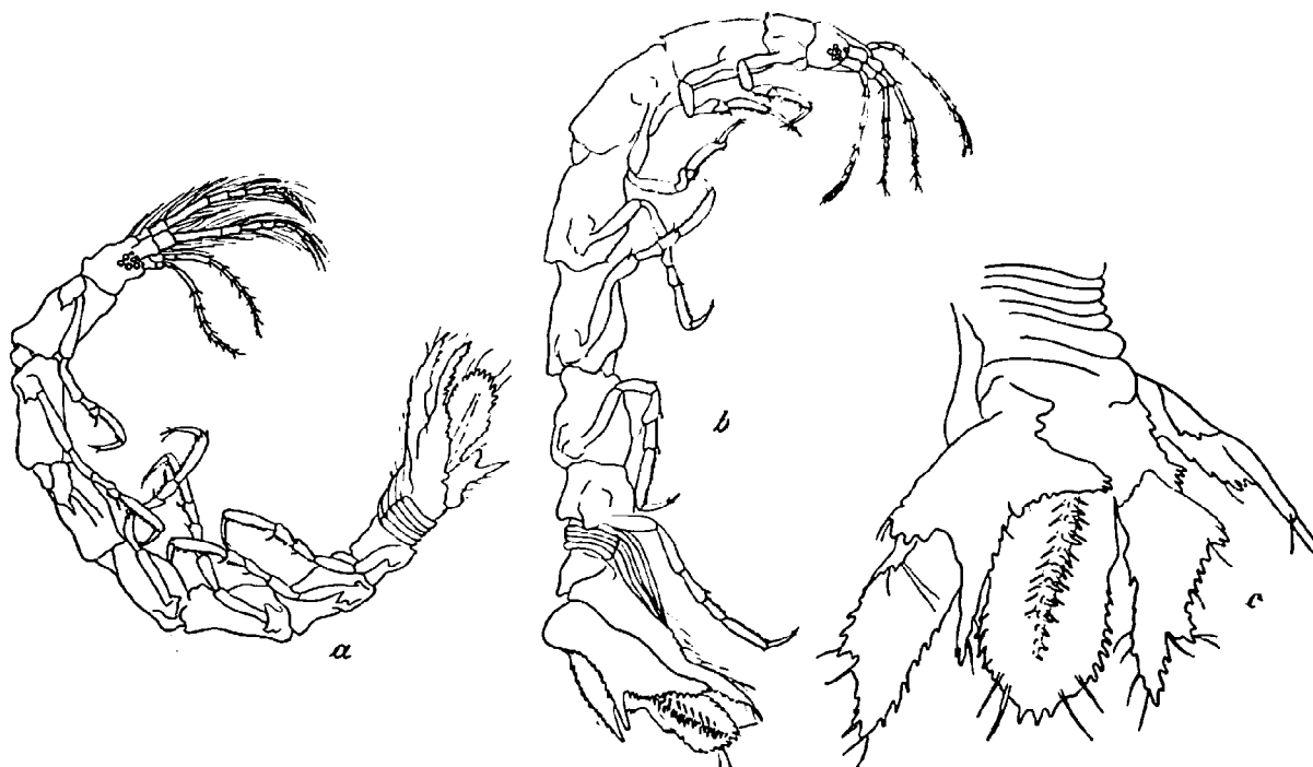
Abb. 33. Eisothistos antarcticus n. sp. a ♂, b ♀ (× 32), c Telson stärker vergrößert.
