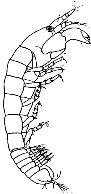
Abb. 13. Leptognathia oculata n. sp. (× 33).
