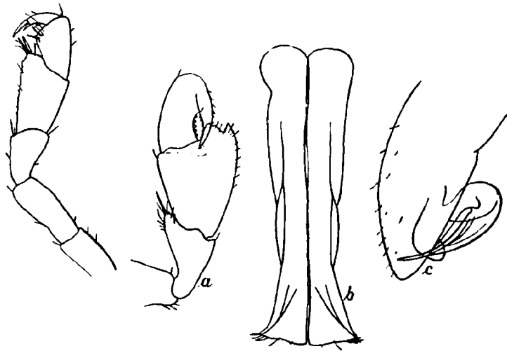
Abb. 97. Munna psychrophila n. sp. a Greiffuß des ♂ ( \times 55 ), b erste, c zweite Pleopoden des ♂ ( \times 70 ).
