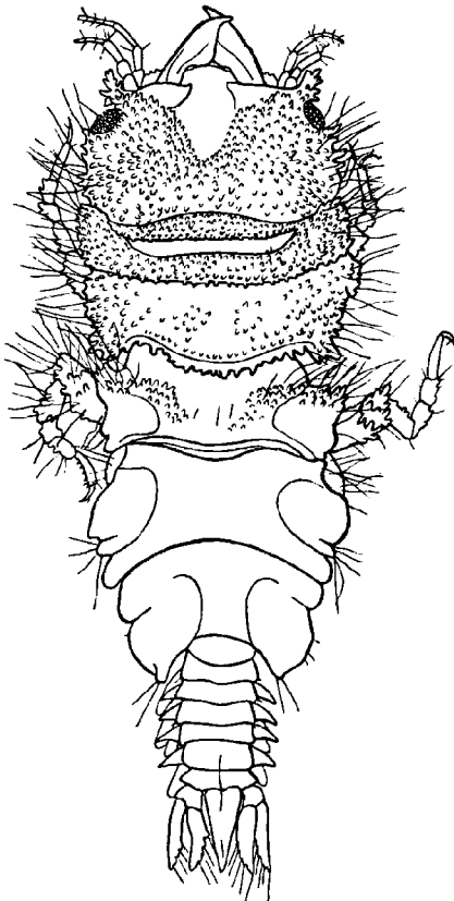
Abb. 25. Gnathia hodgsoni n. sp. ♂ (× 23).
