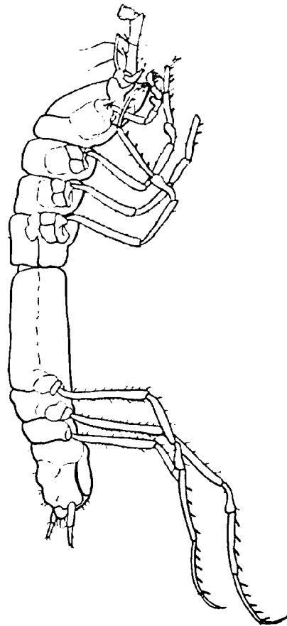
Abb. 88. Rhabdomesus inermis n. sp. (× 18).
