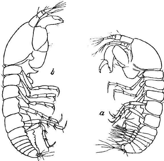
Abb. 19. Cryptocope antarctica n. sp. a ♂, b ♀ (× 36).
