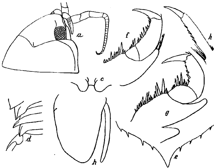
Abb. 36. Cirolana oculata n. sp. a Kopf von der Seite ( \times 4,5 ), b zweiter Pleopod des ♂ ( \times 15 ), c Griffel des ♂ ( \times 10 ), d Seiten der letzten Rumpfssegmente und des Abdomens ( \times 4,5 ), e Spitze der Schwanzplatte ( \times 10 ), f erster Fuß, g zweiter Fuß, h siebenter Fuß ( \times 18 ).
