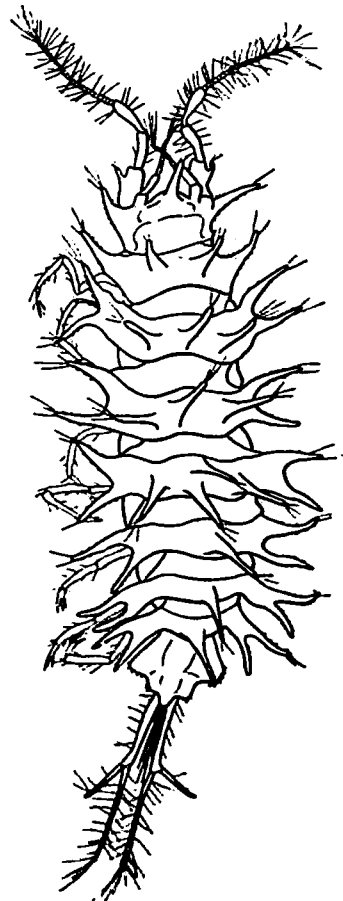
Abb. 67. Janthopsis multispinosa n. sp. ( \times 11 ).
