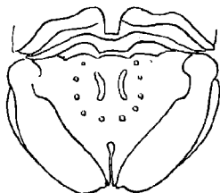
Abb. 47. Cycloidura simpsoni HELLER. Abdomen des ♂ ( \times 6 ).
