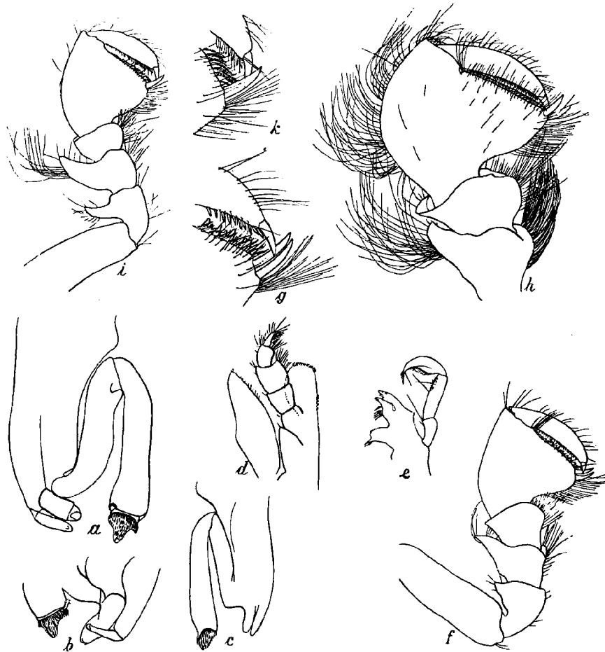
Abb. 73. Stenetrium acutum n. sp. a ( \times 70 ) u. b zweiter Pleopod eines ♂ aus der Tiefsee, c eines ♂ von der Gauss-Station, d Maxillarfuß ( \times 25 ), e Mandibel, f , i Schere des ♀ ( \times 14 ), g , k Zähne derselben, stärker vergrößert ( \times 40 ), h Schere des ♂ aus der Tiefsee ( \times 14 ).
