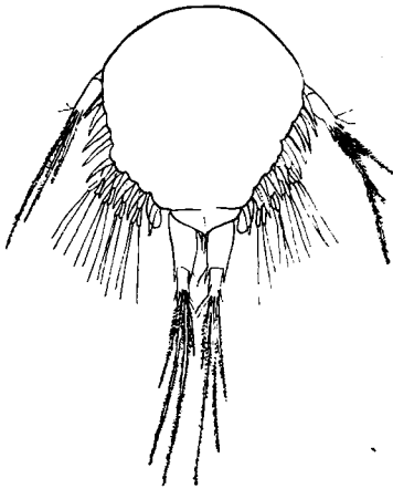
Abb. 132. Cryptoniscus -Larve im ersten Stadium ( \times 167 ).
