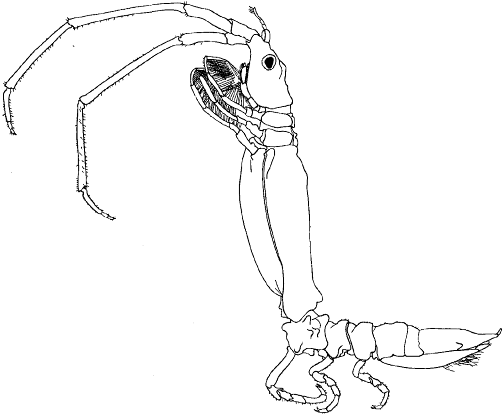
Abb. 54. Astacilla kerguelensis n. sp. ( \times 8 ).
